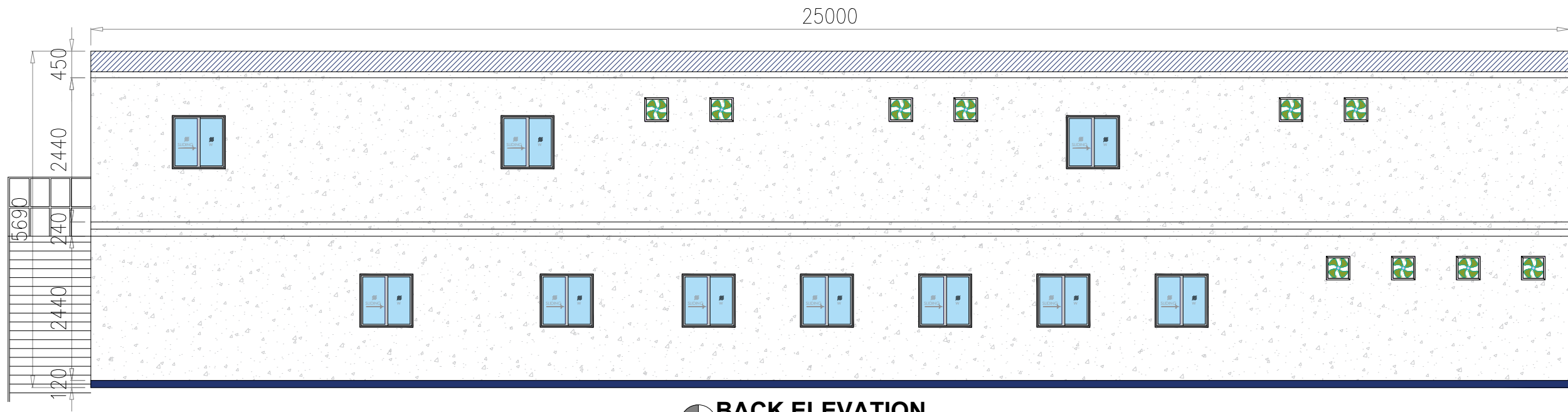
BACK ELEVATION SCALE: 1:40
