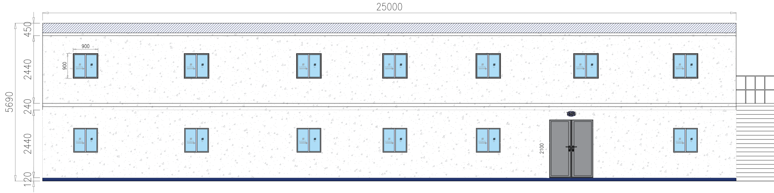
BACK ELEVATION SCALE: 1:40
